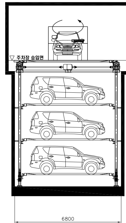
기계식주차장 측면도
