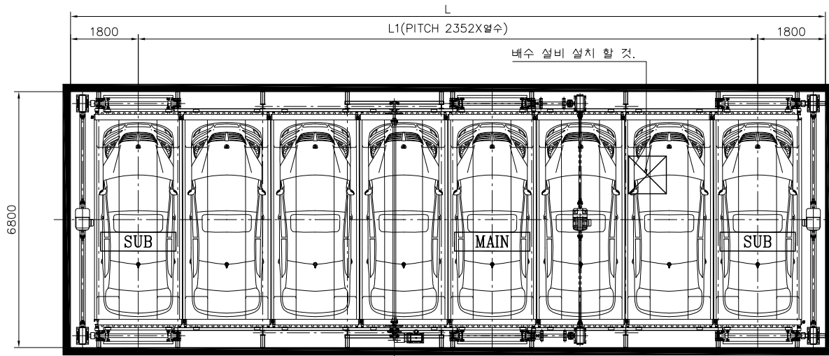
기계식주차장 평면도
