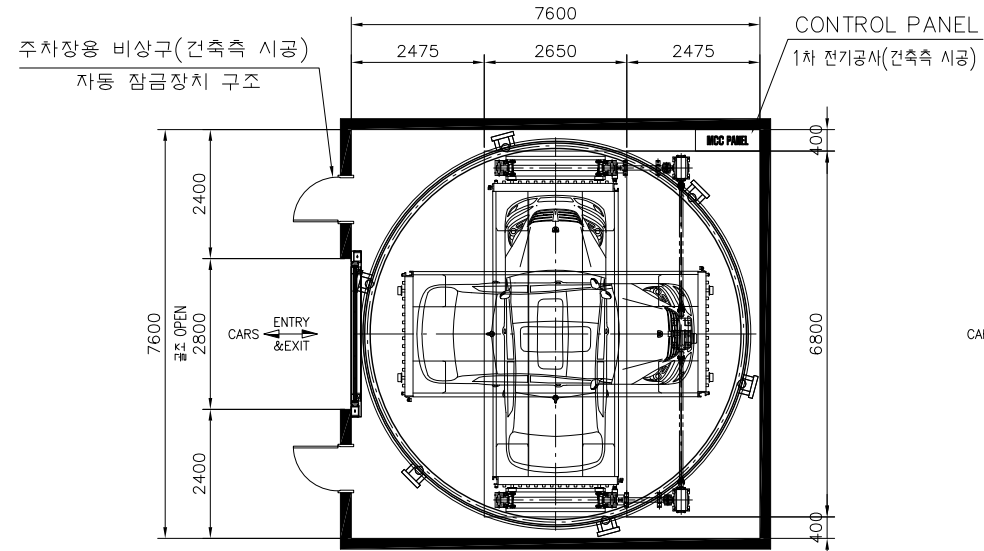
입고층 평면도
