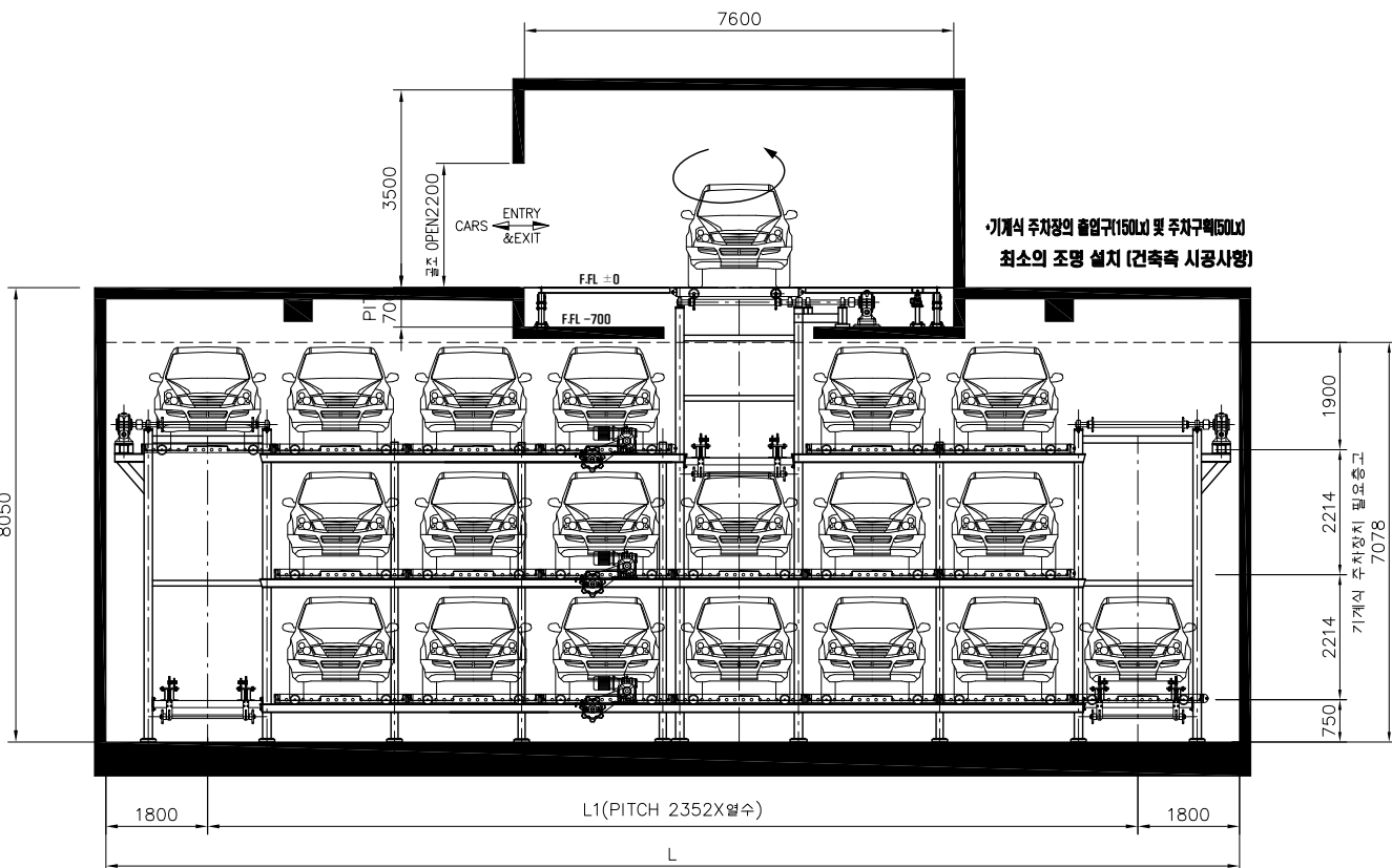
기계식주차장 정면도
