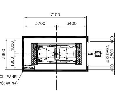
입고층 평면도
