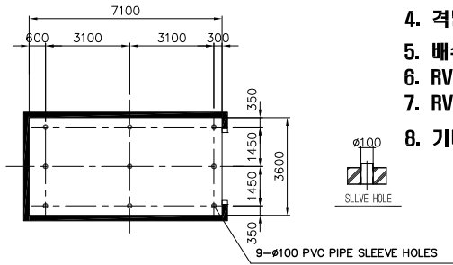
■ SLEEVE HOLE [건축측 시공]
