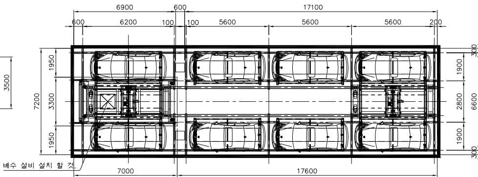
기계식주차장 평면도
