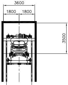
입고층 정면도
