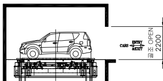
입고층 단면도
