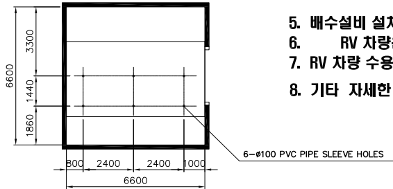
■ SLEEVE HOLE [건축측 시공]
