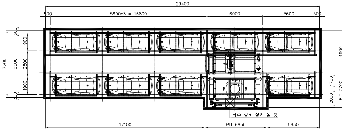
기계식주차장 평면도
