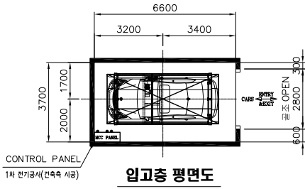
입고층 평면도
