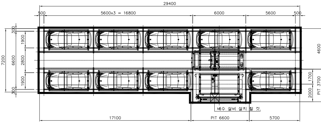
기계식주차장 평면도
