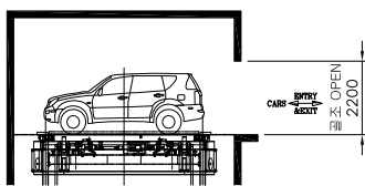
입고층 단면도
