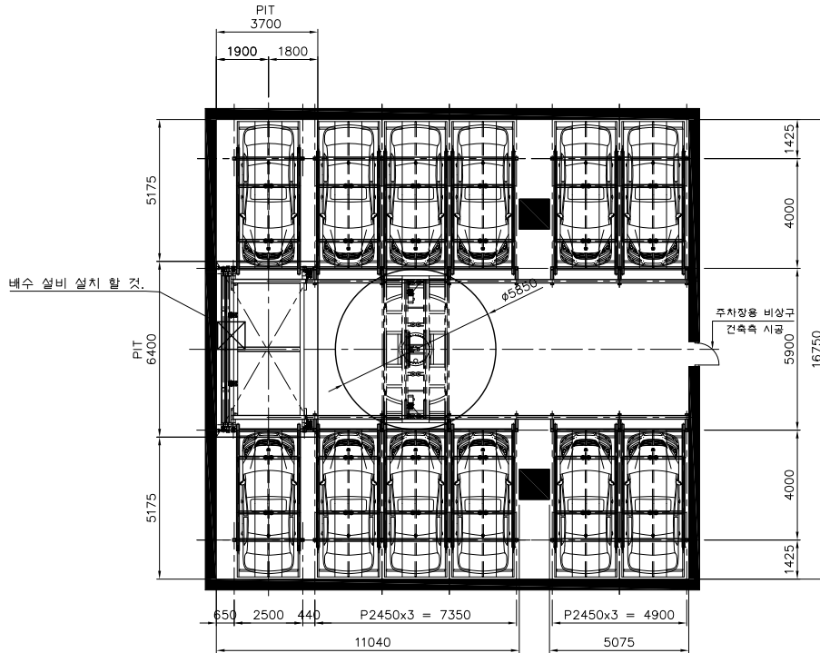
기계식주차장 평면도
