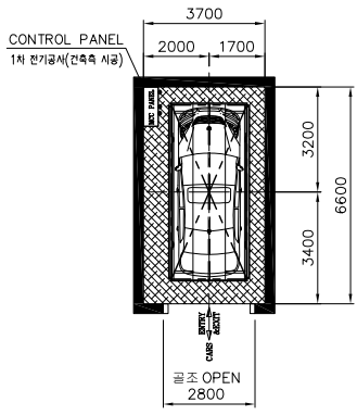
입고층 평면도
