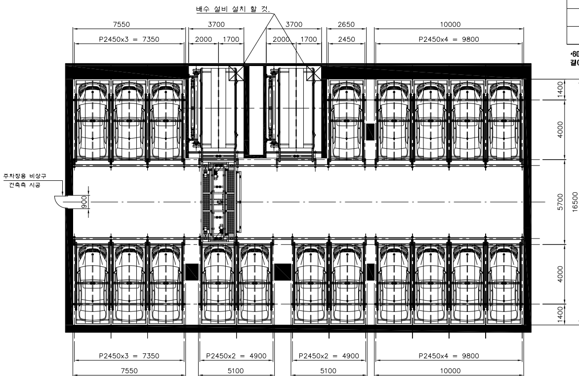
기계식주차장 평면도
