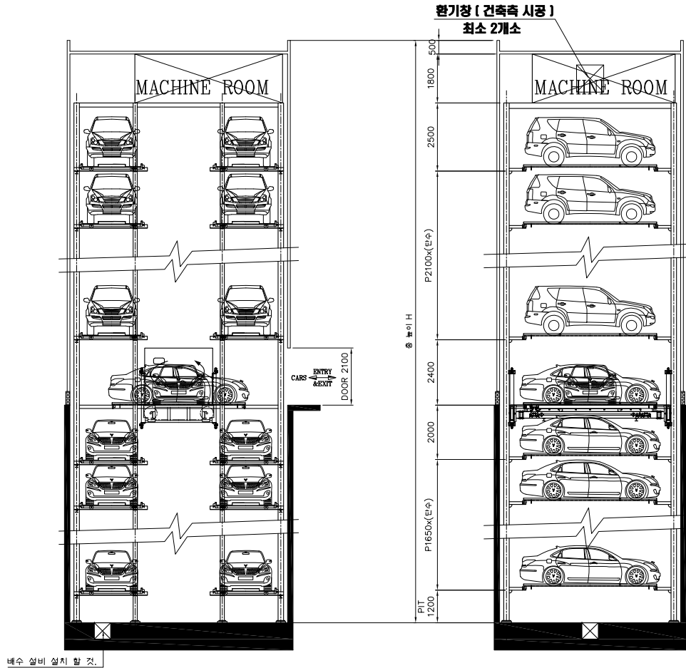
기계식주차장 정면도
