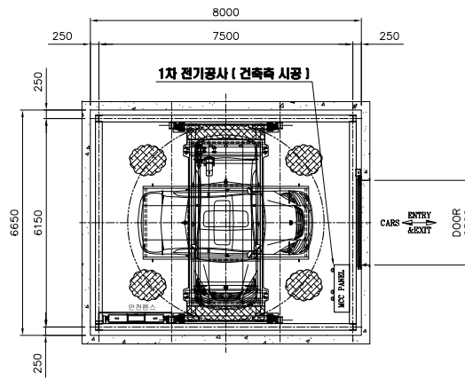
입고층 평면도
