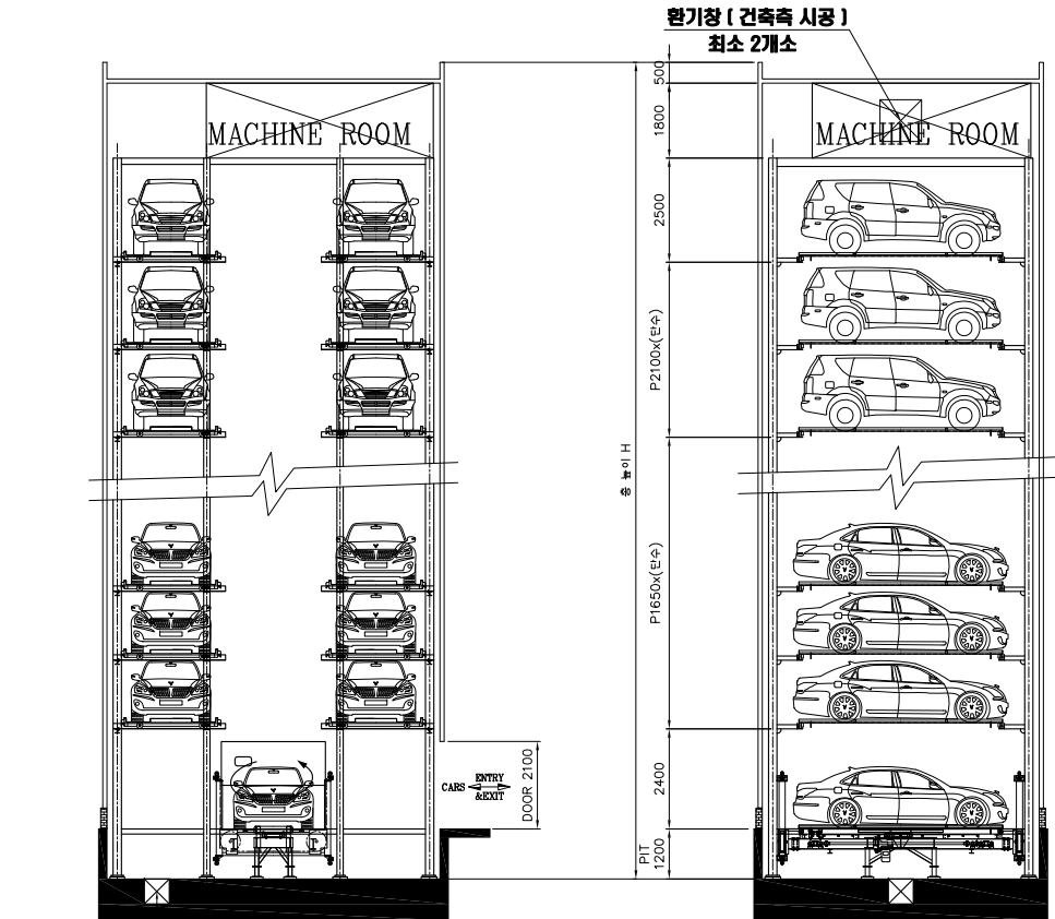
기계식주차장 정면도
