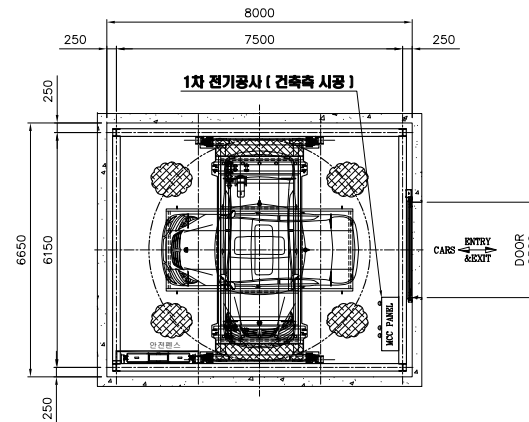
입고층 평면도
